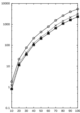
Fig. 12. gas, prop. 3, l2s
